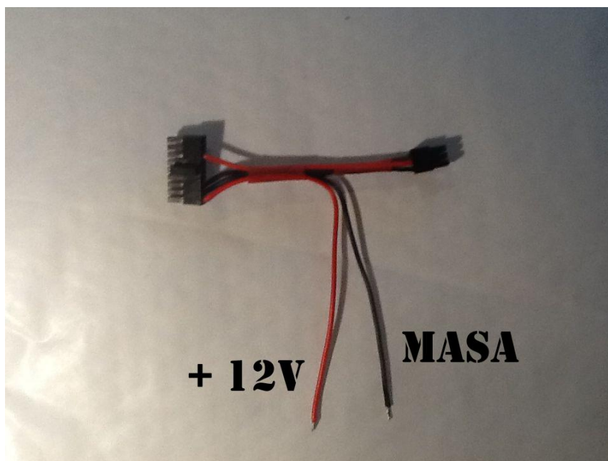
Wiązka mL300-S5-1
