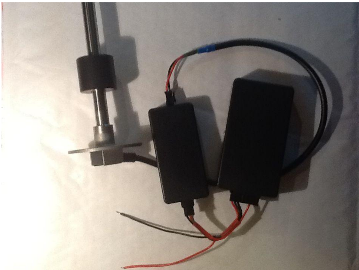
Kompletna instalacja
